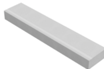
מדרגת המרינה AC-64-33 160X33X15 AC-64-40 160X40X15
