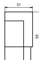
מדרגת ישיבה פינה חיצונית RG-43OUT 31X31X55
