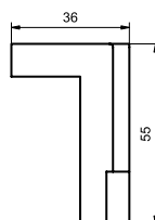
מדרגת ישיבה פינה פנימית RG-43IN 36X36X55
