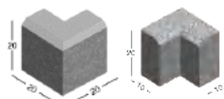
אבן גן פינה חיצונית MS - 4A אבן גן פינה פנימית MS - 4A1 10X20X20 ס"מ
