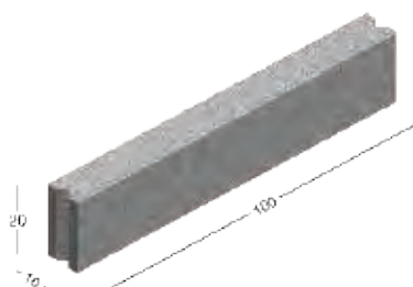
אבן גן ללא פאזה MS - 4-1 10X20X100 ס"מ
