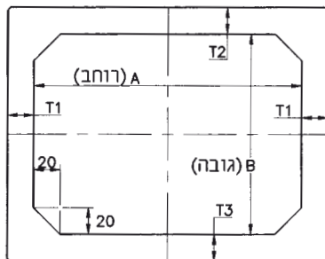
פרט חבור שקע תקע בין היחידות
