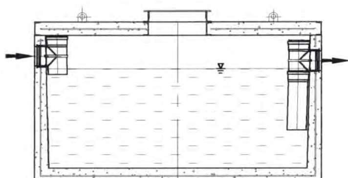
מפריד שומנים אורגניים GREASE SEPARATOR
