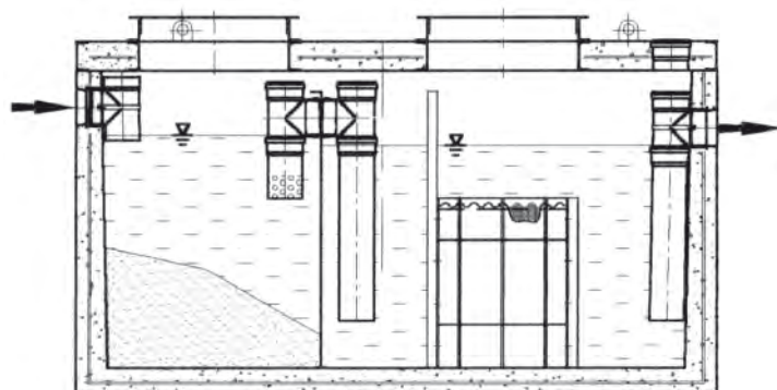
מפריד שמנים ודלקים מינרליים משולב עם מיכל שיקוע
