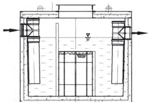
מפריד שמנים ודלקים מינרליים COALESCENCE SEPARATOR
