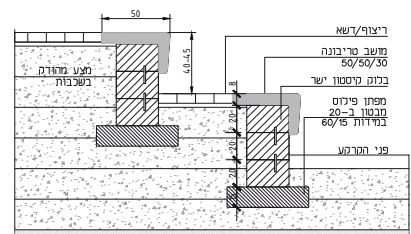
טריבונה על גבי טרסות מבלוקי קיסטון
